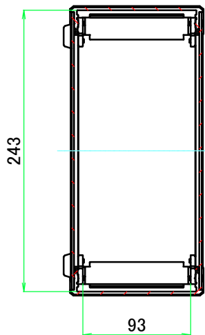
A-A ( 1 : 4.5 )
