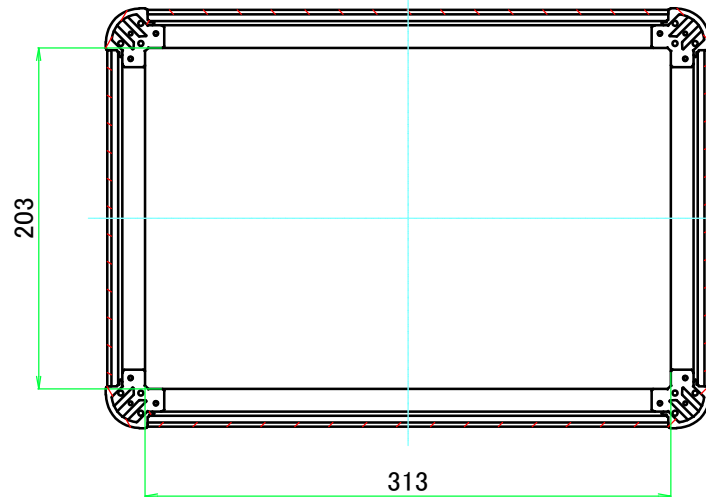
C-C ( 1 : 4.5 )
